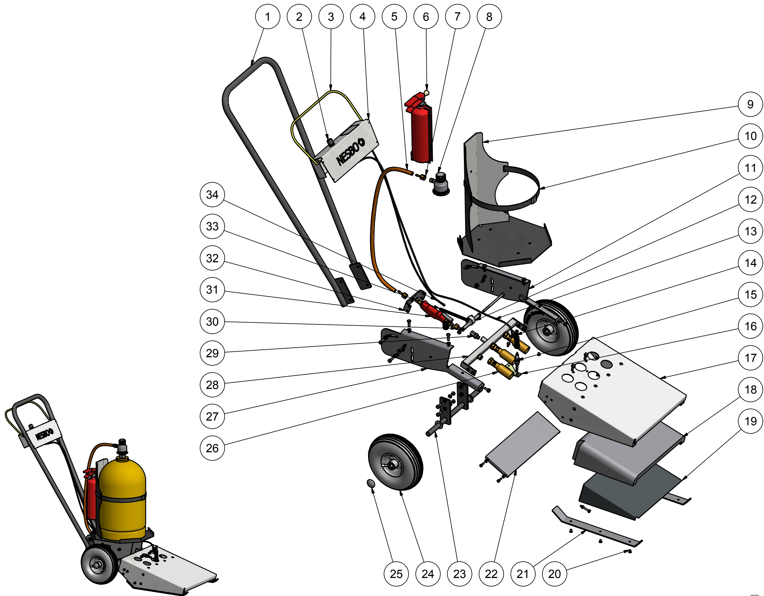
Ukrudtsbrænder GF 350 A
